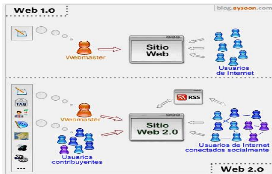
Ilustración 9: La web 2.0
