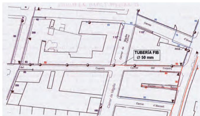
Figura 2: Tubería de fibrocemento
