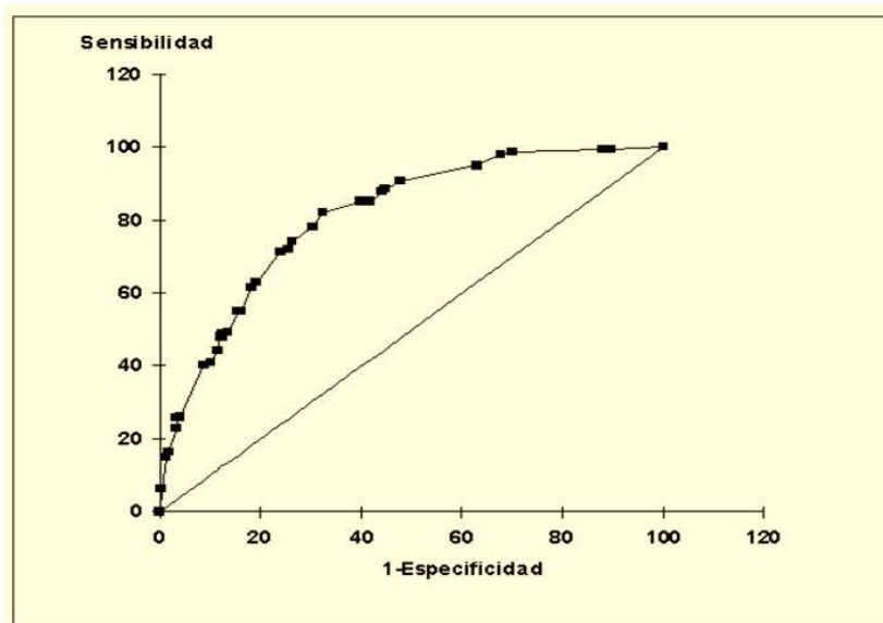
Figura 6. Curva ROC
